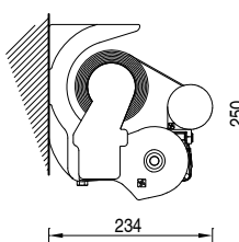
Installation façade avec support façade/plafond
