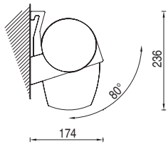
Installazione a parete 80° 80° wall installation
