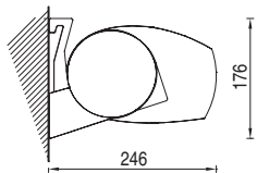
Installazione a parete Wall installation
